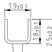
剖面 C-C
