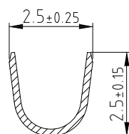
剖面 A-A
