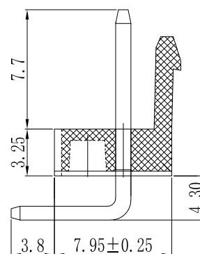
SEC: A-A
